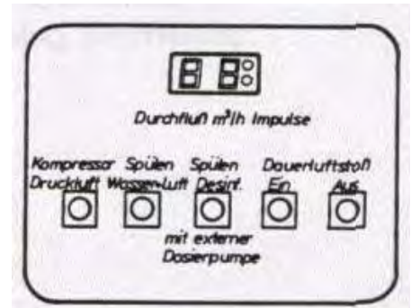
Панель обслуживания
