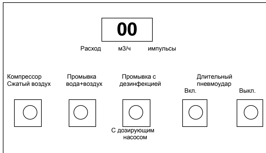
Панель обслуживания
