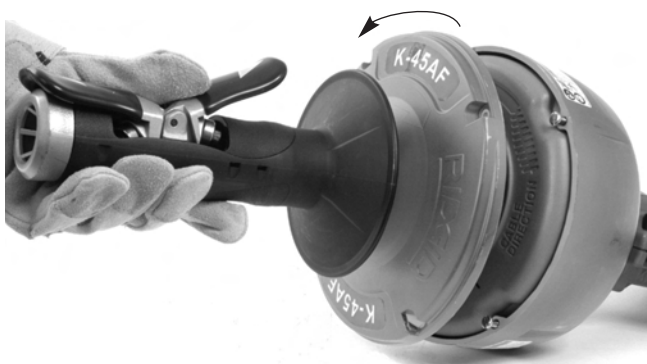
Figure 14 – Ouverture du tambour
