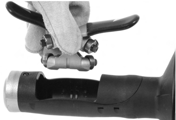
Figura 12B – Extracción del mecanismo de la AUTOFEED
