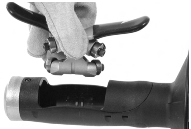
Figura 12B – Demontarea mecanismului AUTOFEED din carcasă
