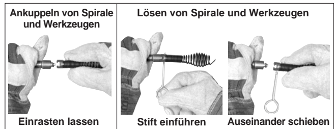
Abbildung 7 – Anschließen und Lösen von Werkzeugen
