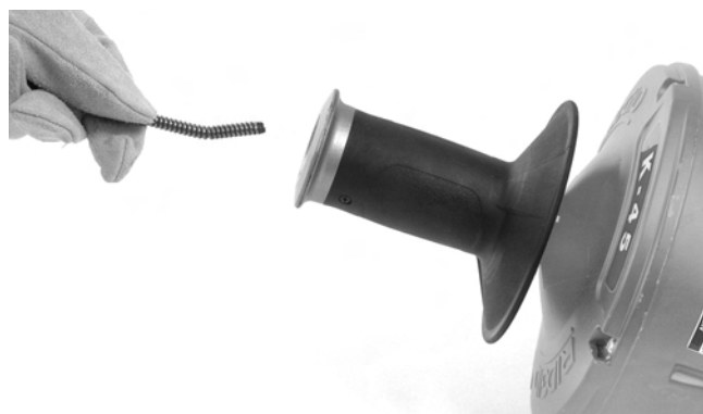
Slika 17 – Vstavljanje kabla brez menjave notranjega bobna
