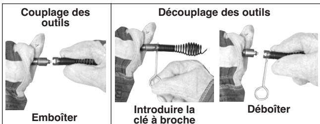
Figure 7 – Couplage et découplage
