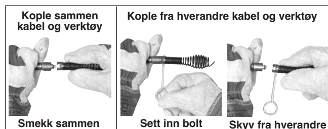
Figur 7 – Tilkopling og frakopling av verktøy
