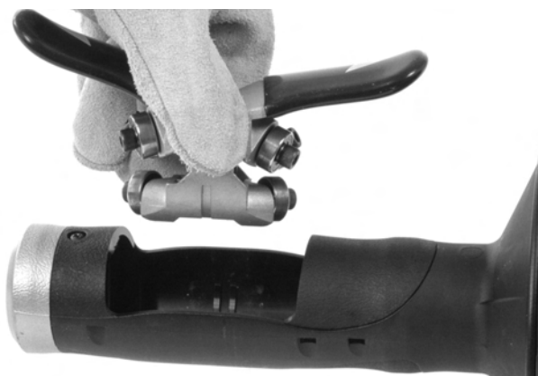
Slika 12B – Skidanje AUTOFEED mehanizma sa kućišta
