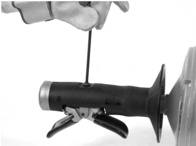
Figura 12A – Rimozione della vite AUTOFEED
